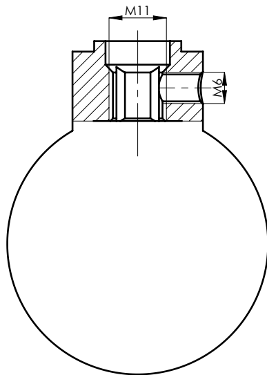
SEZIONE A-A
