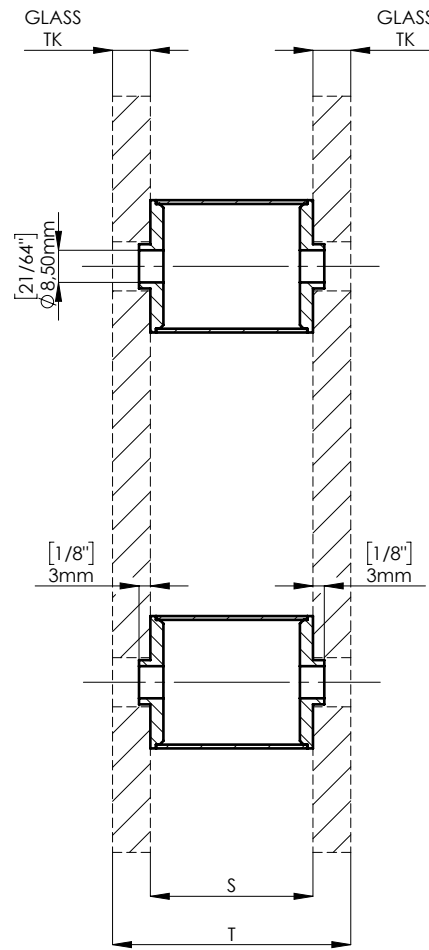
SECTION A-A
