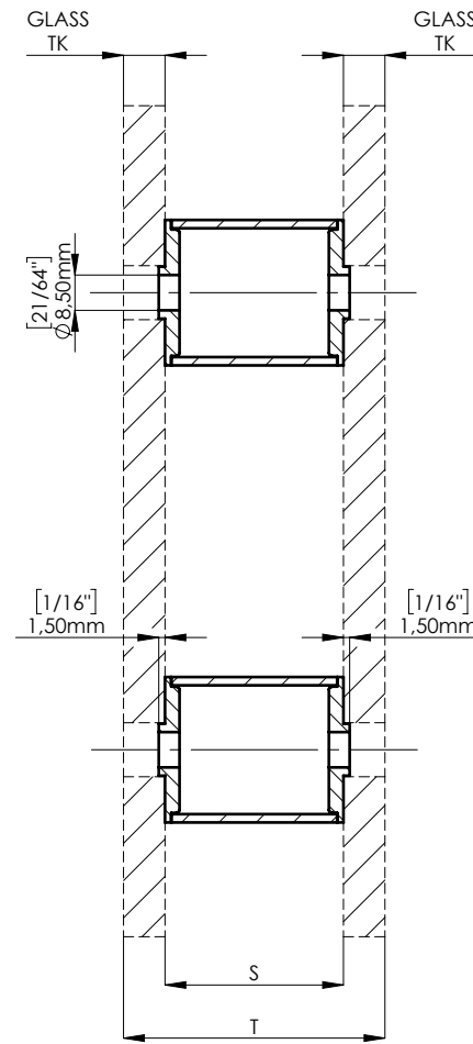
SECTION A-A
