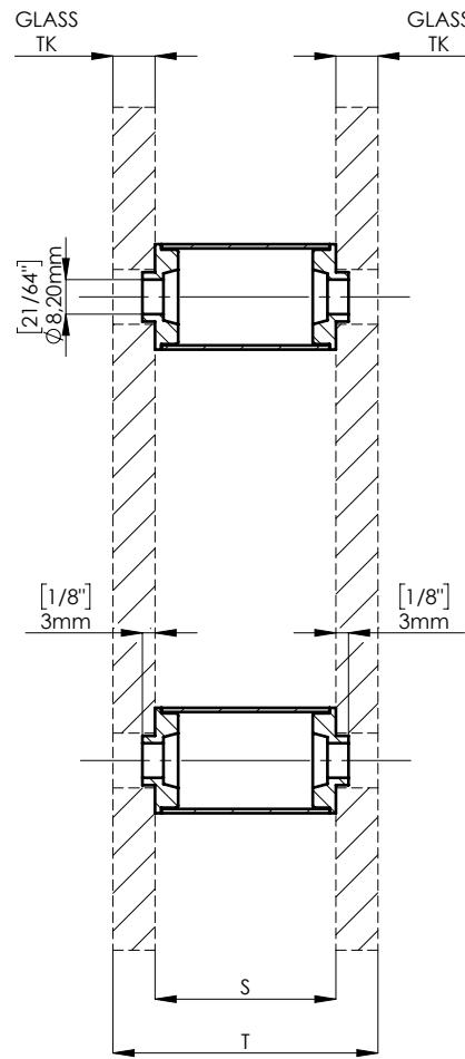
SECTION A-A
