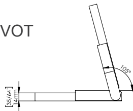
OUVERTURE MAXIMALE
