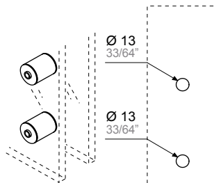
ITEM 2AT.KIT.9905 2AT.KIT.9907 2AT.KIT.9909 Ø 25 mm 30 mm 35 mm
