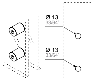
ITEM 2CC.KIT.0005 2CC.KIT.0007 2CC.KIT.0009 Ø 25 mm 30 mm 35 mm
