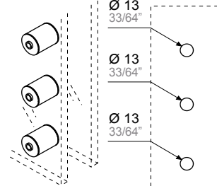
ITEM 2AT.KIT.9906 2AT.KIT.9908 2AT.KIT.9910 Ø 25 mm 30 mm 35 mm
